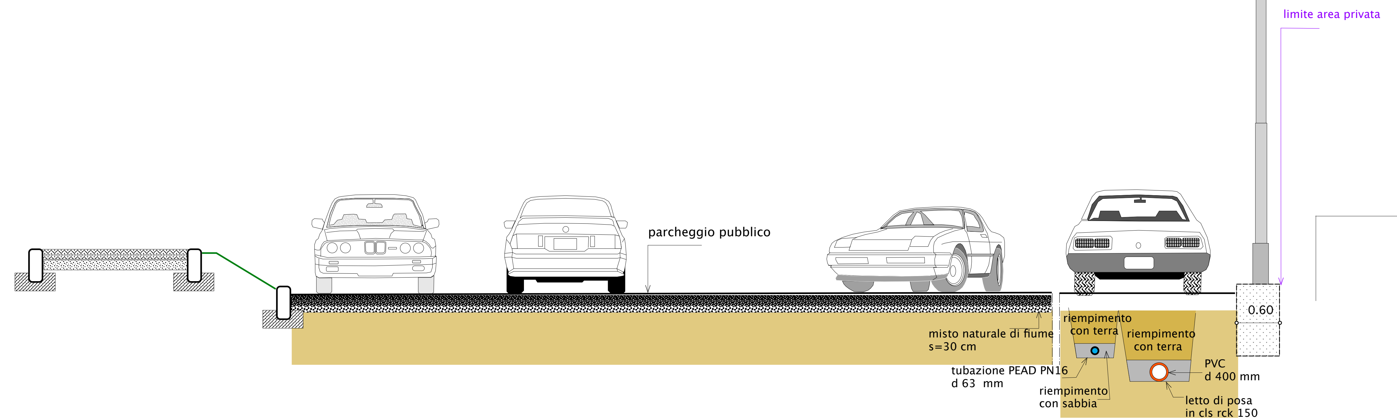
sezione tipo piazzale marciapiede
