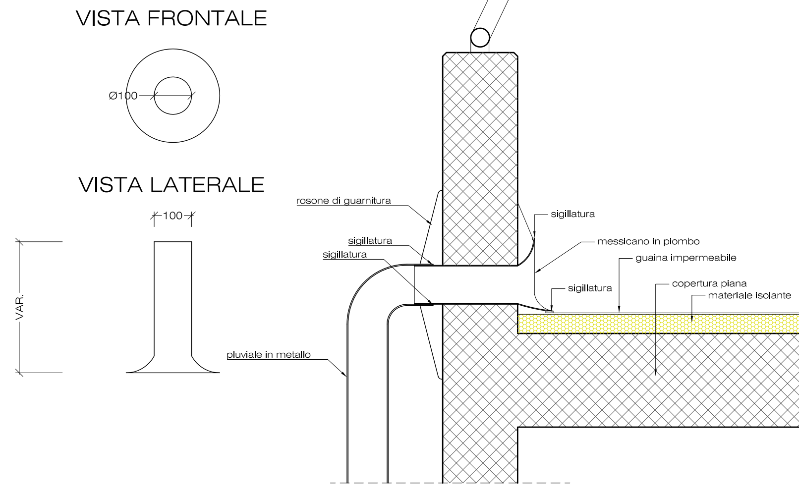
MESSICANI RACCOLTA ACQUE METEORICHE PARTICOLARE COSTRUTTIVO Scala 1:10
