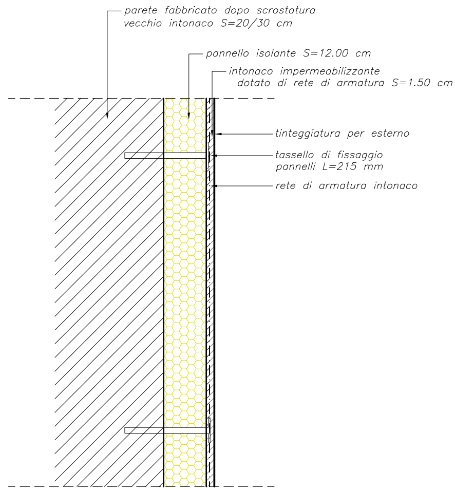
COIBENTAZIONE ESTERNA FACCIATA PARTICOLARE COSTRUTTIVO Scala 1:10
