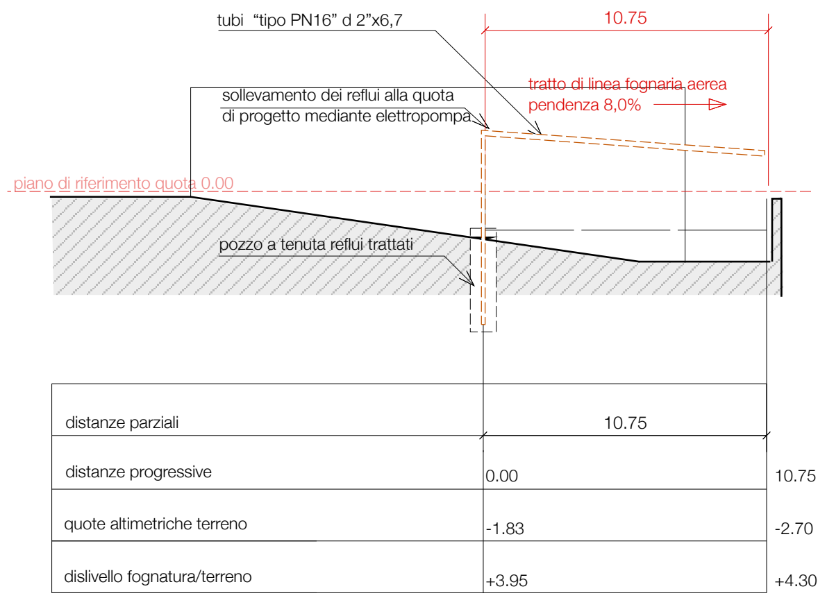
sezione b - profilo longitudinale scala 1:200
